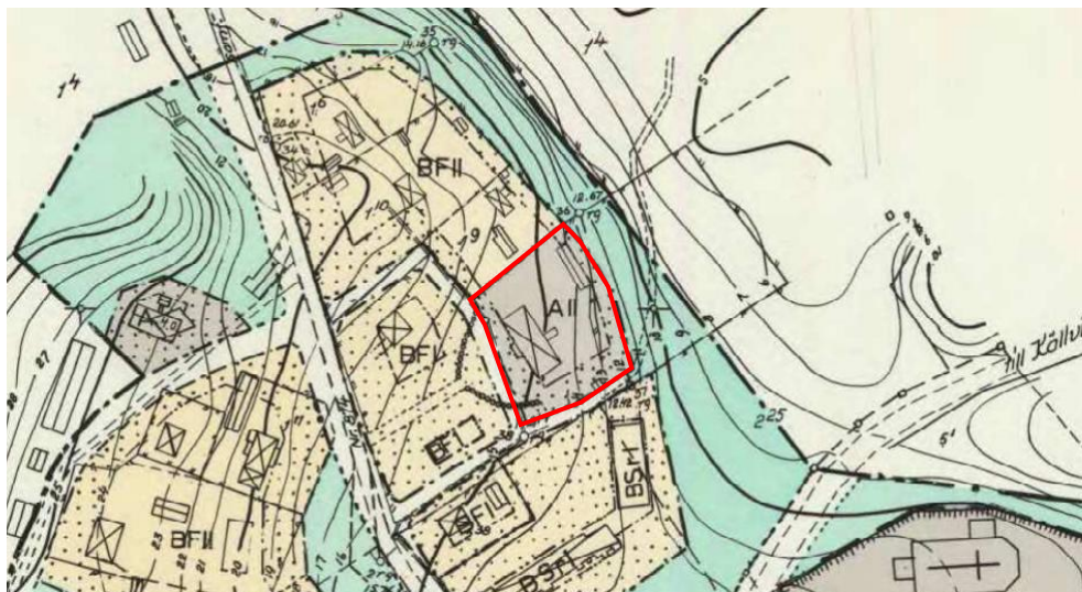
Figur 8. Förslag till byggnadsplan för område vid Tångered i Loftahammar socken och kommun. Berörd del markerad med röd linje.
