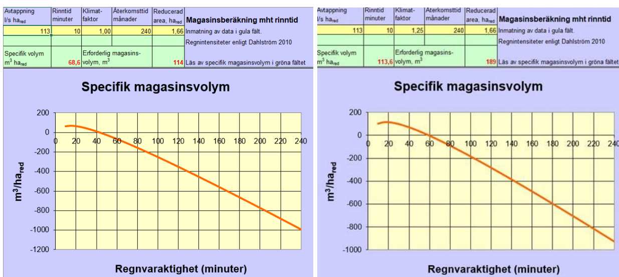
Diagram ur P110 bilaga 6a visande volymbehov utan och med klimatfaktor pålagd.
