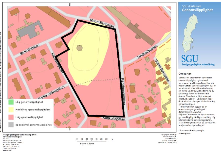
Figur 7. Skattade genomsläpplighet inom planområdet, enligt SGU. Svart linje visar ungefärlig plangräns. © Lantmäteriet.
