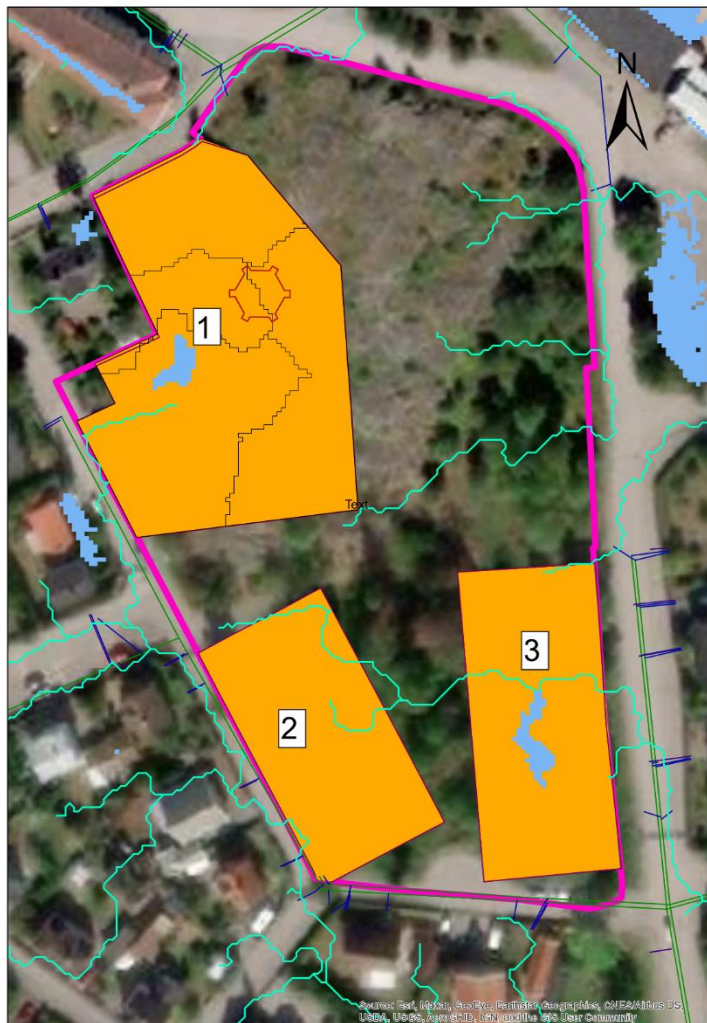
Figur 13. Illustration av sänkor (blått) inom kvarteren (orange) som riskerar att översvämmas vid skyfall. Hämtat från Scalgo Live. © Ortofoto från ArcMap
