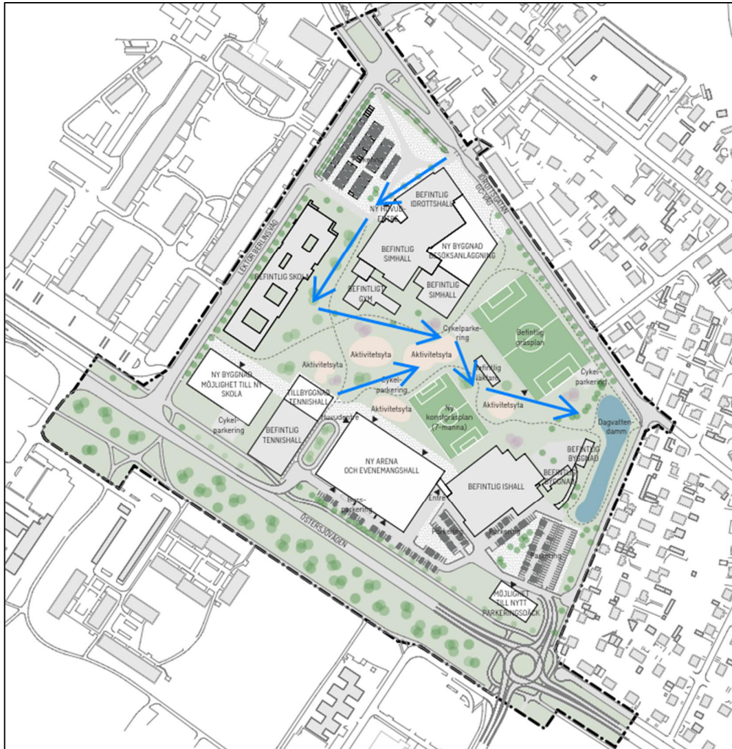
Figur 30. Blå pilar visar exempel på placering av dikesstråk genom planområdet som kan breddas ut på aktivitetsytor vid framtida skyfallsregn.
