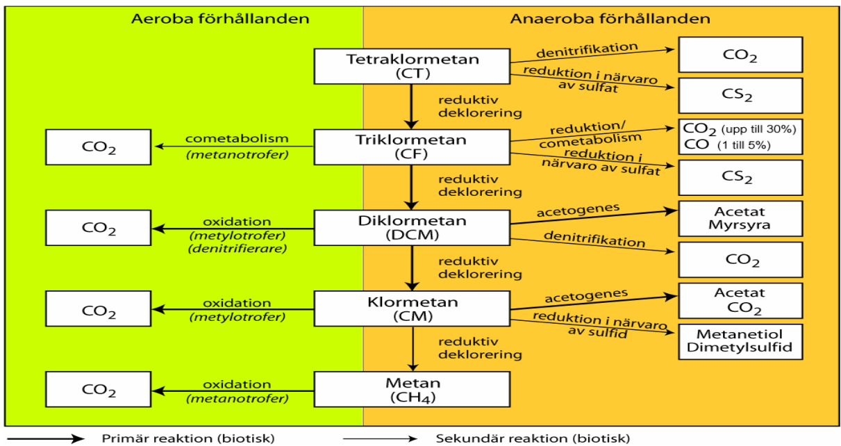
Figur 14. Nedbrytningsvägar för klormetaner (Figur 3.8 ur NV 5663, Hållbar Sanering, 2007); "Klorerade lösningsmedel..."
