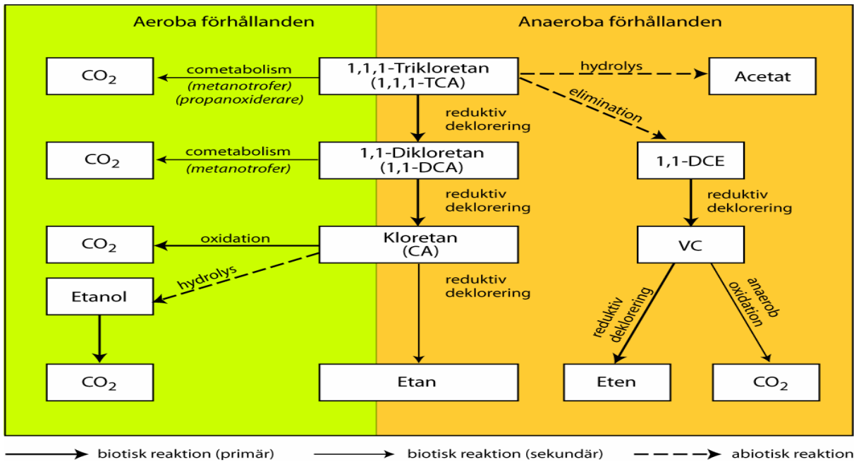
Figur 13. Nedbrytningsvägar för 1,1,1-TCA (Figur 3.7 ur NV 5663, Hållbar Sanering, 2007); "Klorerade lösningsmedel..."
