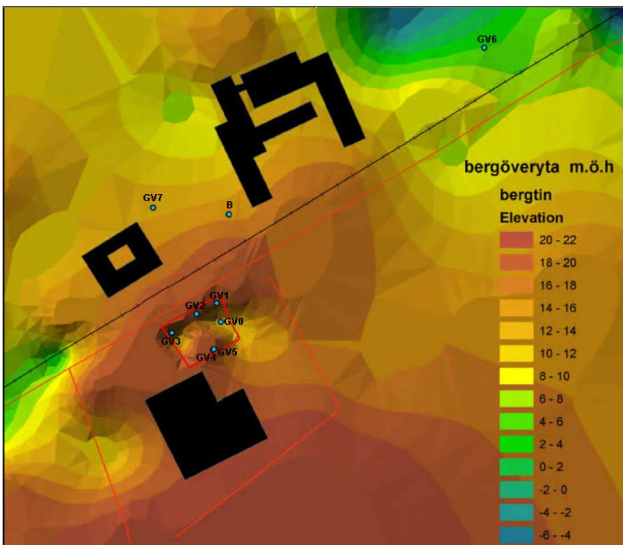
Figur 3: Uppmätt djup till berg (modell efter Meland 2001, grafik A Svensson) Bild hämtad från Förstudie 2009, Västerviks kommun
