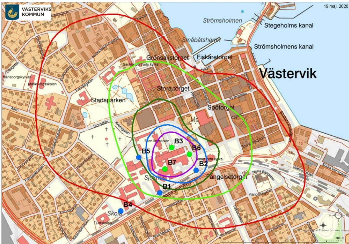
Figur 10 . Influensområde, påverkan av grundvattennivåer vid vattenuttag från grv.rör/ borrhål B3, B6, B7 borrhål/ brunnar för grundvatten. B3, B6, B7 är platser för uttag av reservvatten (gröna punkter) grv-rör B1, B2, B4, B5 för provtagning-kem.analysis (blå punkter).
