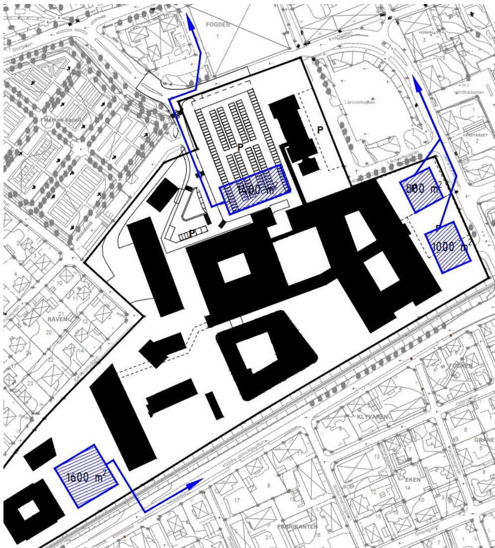
Figur 19. Förslag på placering av dagvattenanläggningar under etapp 10 (avslutande utbyggnad enligt LOST)
