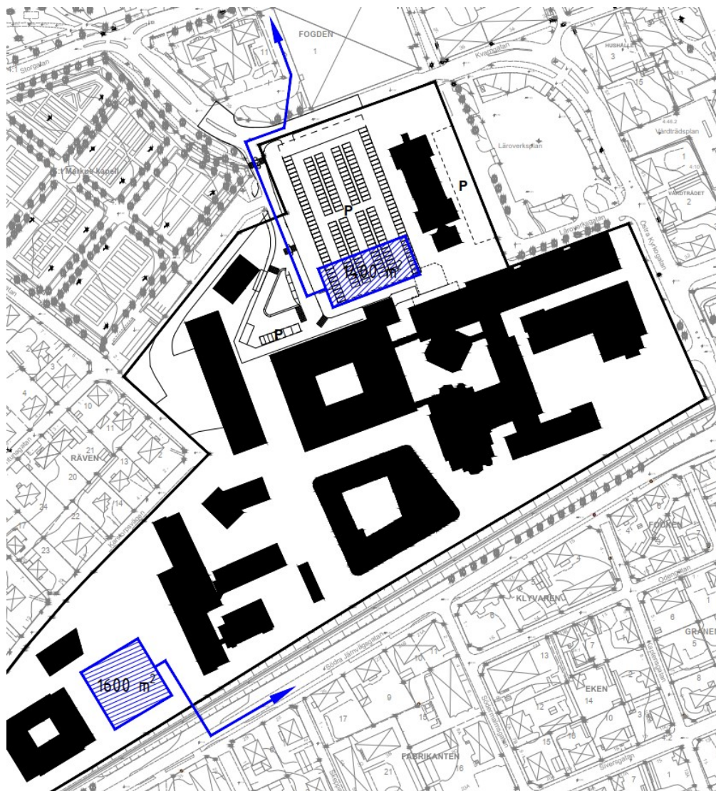
Figur 17. Förslag på placering av dagvattenanläggningar under etapp 5.
