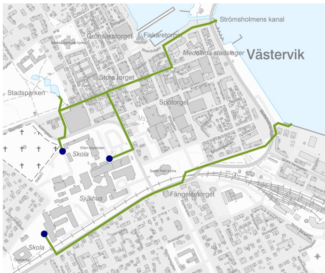
Figur 12. Figuren visar kommunala dagvattenledningar från planområdet och till dess utlopp i havet (gröna linjer). Anslutningspunkterna till planområdet är markerade som blå punkter.
