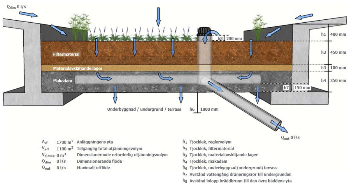
Figur 20. Principskiss på regnbädd (StormTac). Där högre halt föroreningar förekommer i marken sker tätning med duk.
