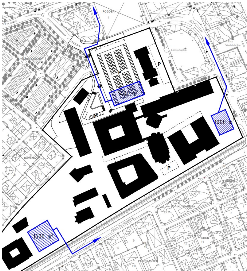
Figur 18. Förslag på placering av dagvattenanläggningar under etapp 7 .
