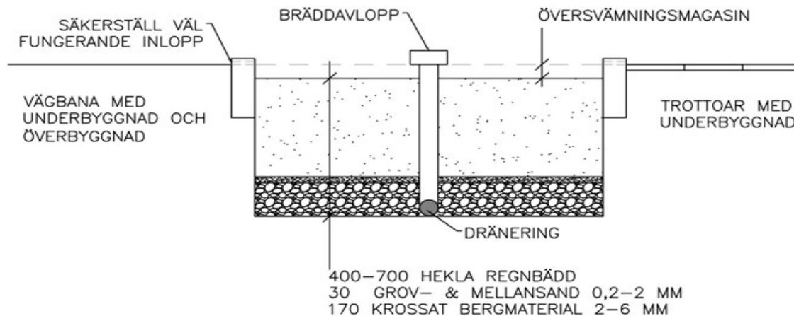
Figur 22. Principlösning för nedsänkt regnbädd. Regnbäddens uppbyggnad består av tre skikt. En översvämningsszon som kan svämma över vid extremväder, en buffertzon som ska fördröja lagra och/eller ta upp vatten under längre tid. I botten ett dräneringslager. Referens: Figur hämtad från www.baramineraler.se
